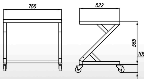
СХЕМА ПОДСТАВКИ
