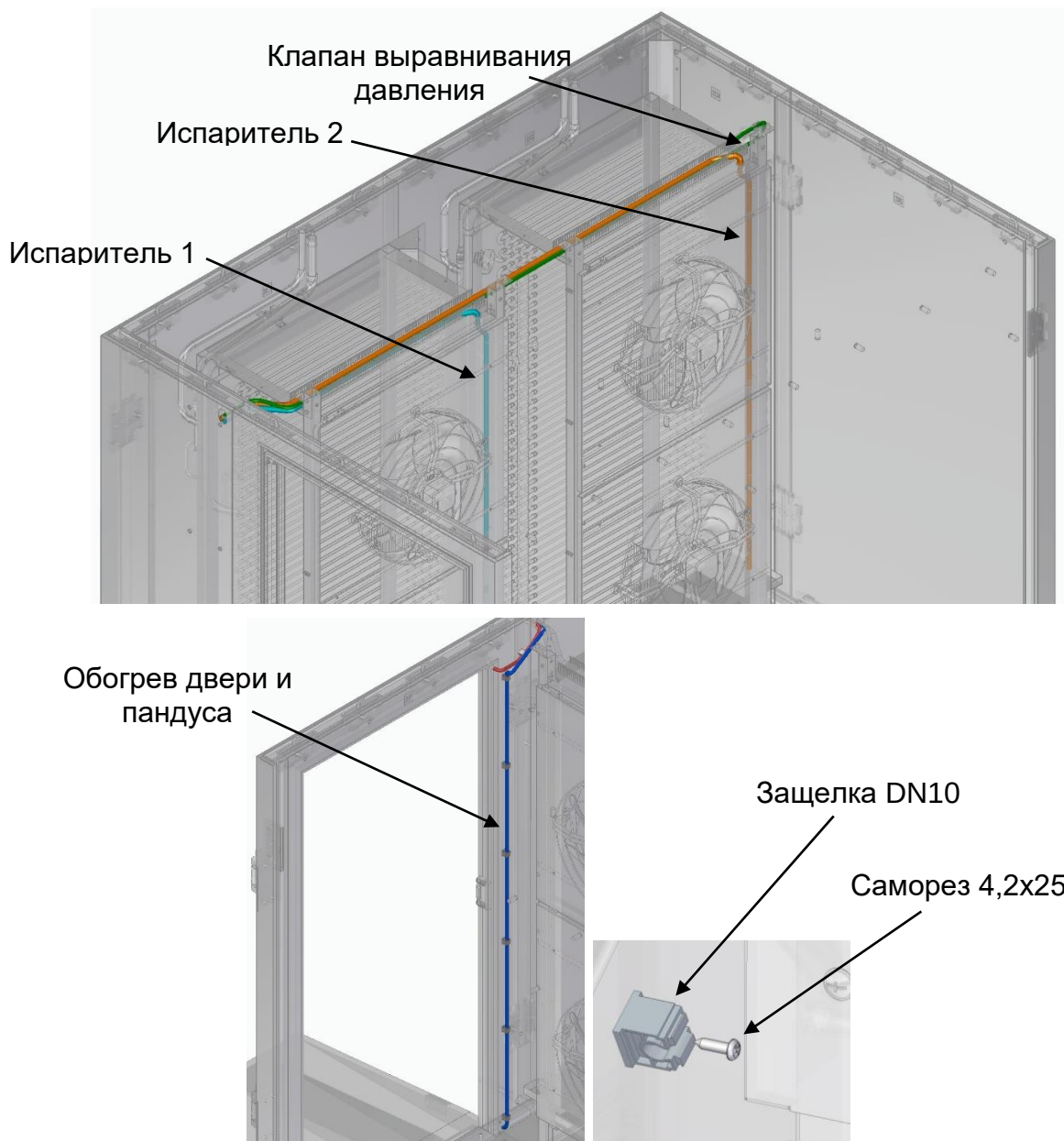
Рис. 18 Укладка проводов
