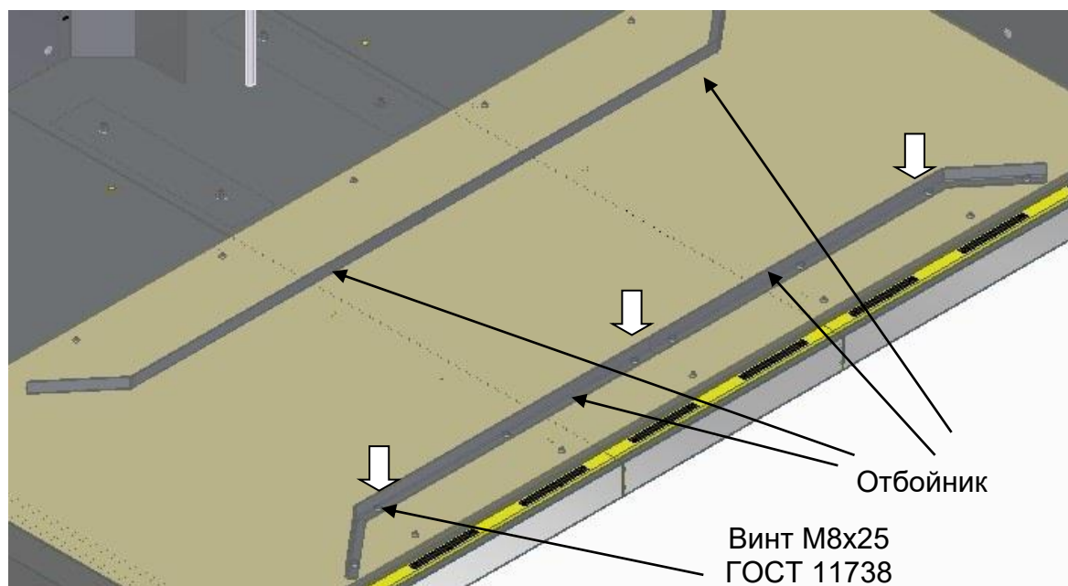
Рис. 26 Установка отбойника
