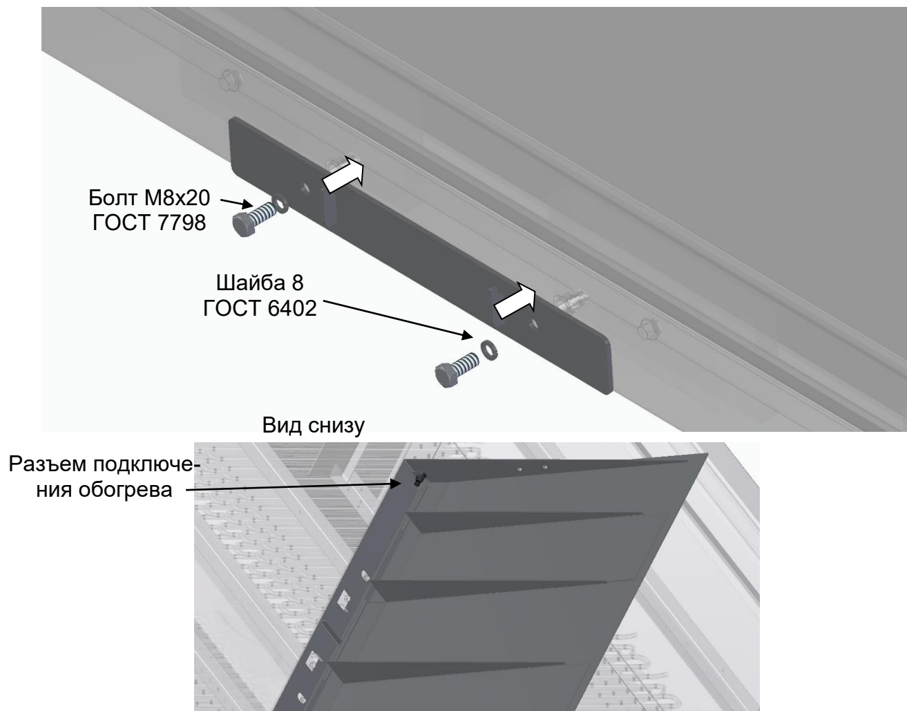
Рис. 25 Установка пандуса
