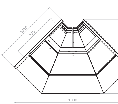
Внутренний угол (динамическое охлаждение)
