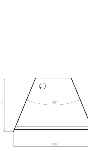
Прилавок внешний угол
