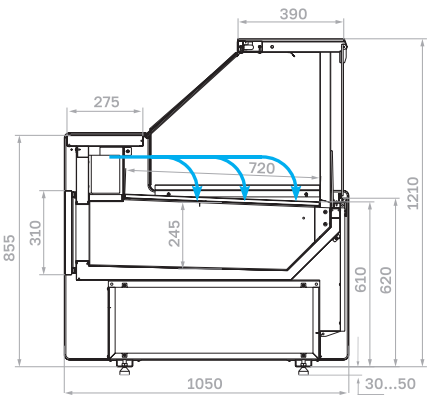
Статическое охлаждение
