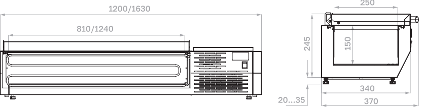
A30 SM 1,2 с крышкой (5 GN1/4)
