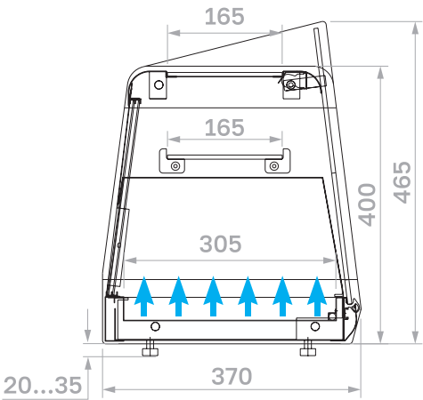
Статическое охлаждение
