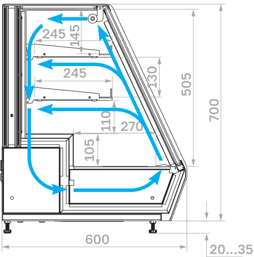
Динамическое охлаждение
