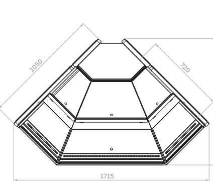
Внешний угол (динамическое охлаждение)
