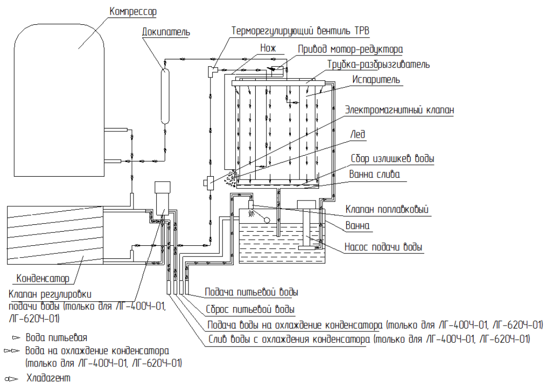
Рис.4 Режим заморозки
