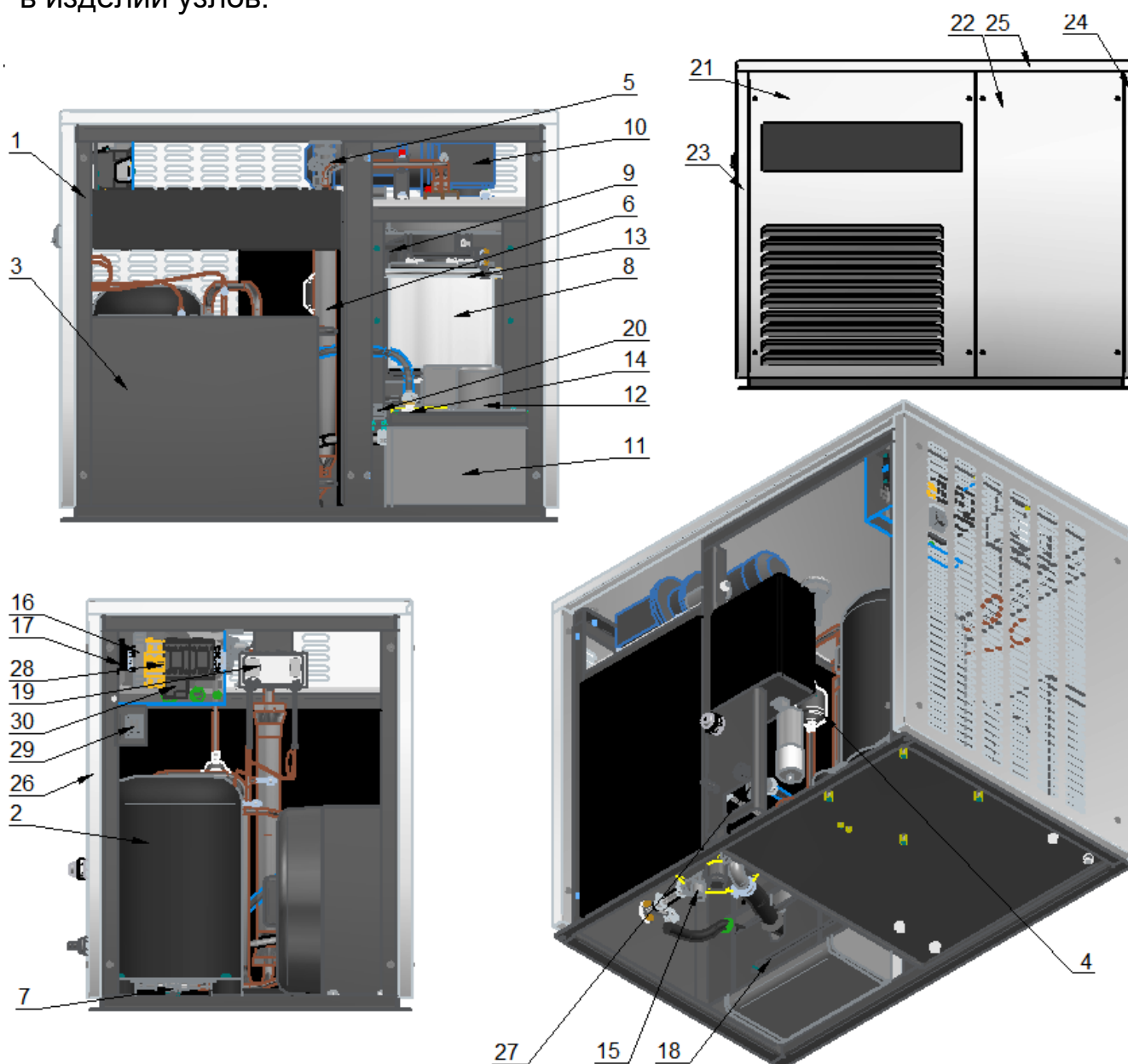
Рис. 2 Устройство льдогенераторов ЛГ-250Ч-02, ЛГ-400Ч-02, ЛГ-620Ч-02
