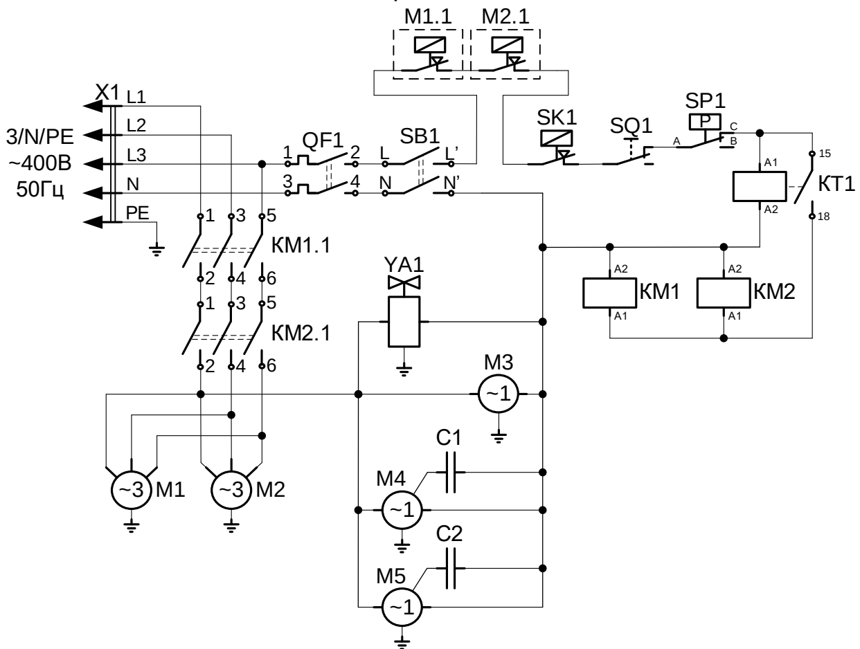
Рис 11. Схема электрическая соединений ЛГ-620Ч-01
