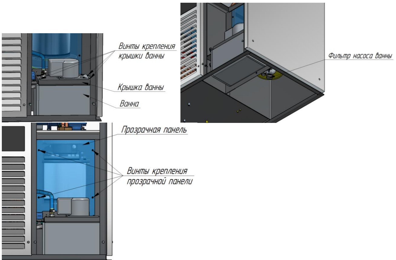
Рис. 8 Расположение крышки ванны, фильтра насоса и прозрачной панели. Смотровая панель на рис. 8 не показана.
