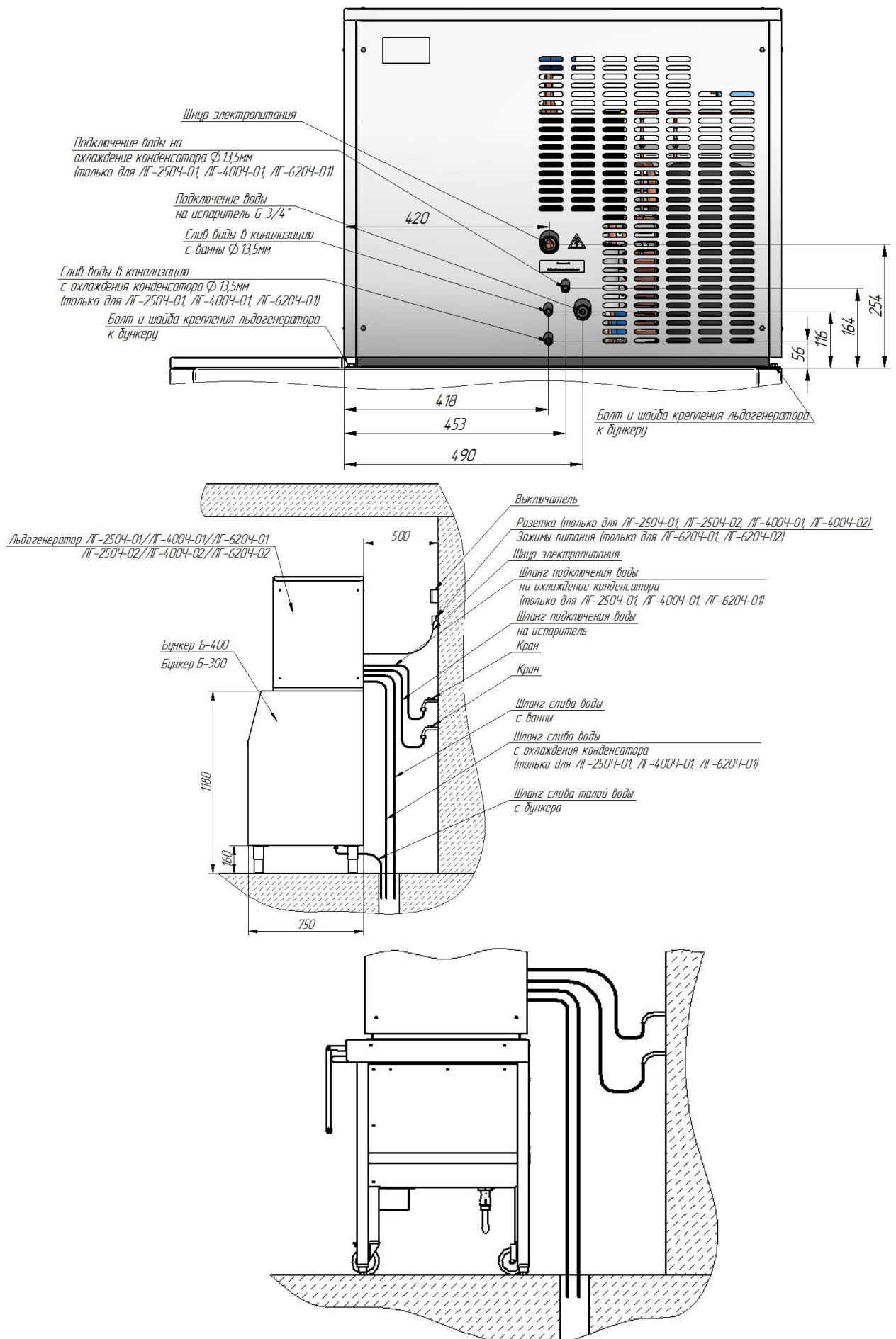
Рис. 5 Схема подключения льдогенератора (с бункером Б-300 или Б-400 и бункером-накопителем БН-2-100)
