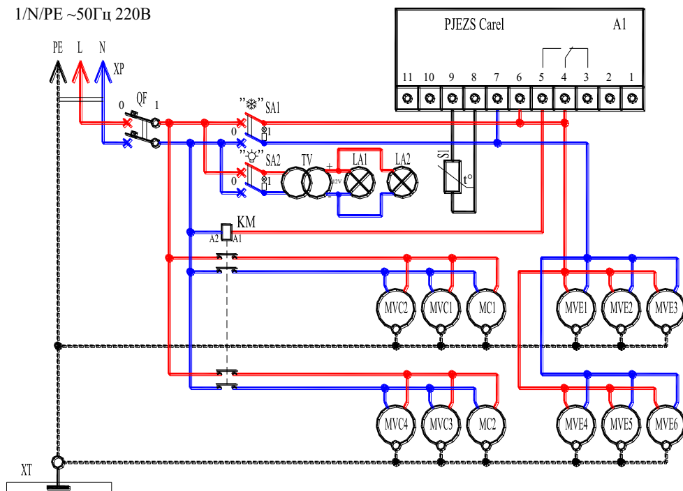
Рис.4. Схема электрическая принципиальная витрины холодильной Carboma 1930/710 ВХСп-2,5. 1/Н/РЕ ~50Гц 220В
