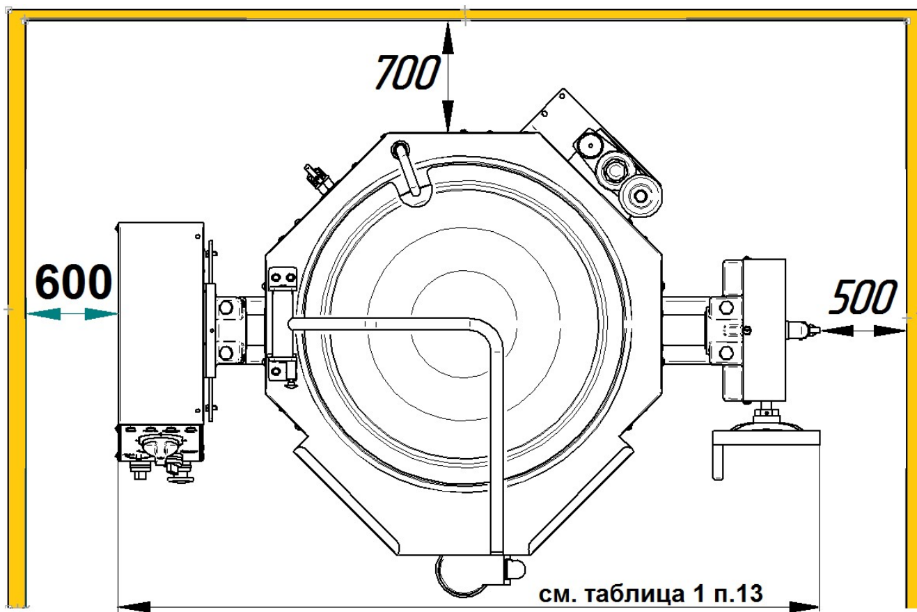
Рис. 3. Установка котла
