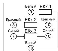
Схема выводов ТЭНа EK1, EK2.
