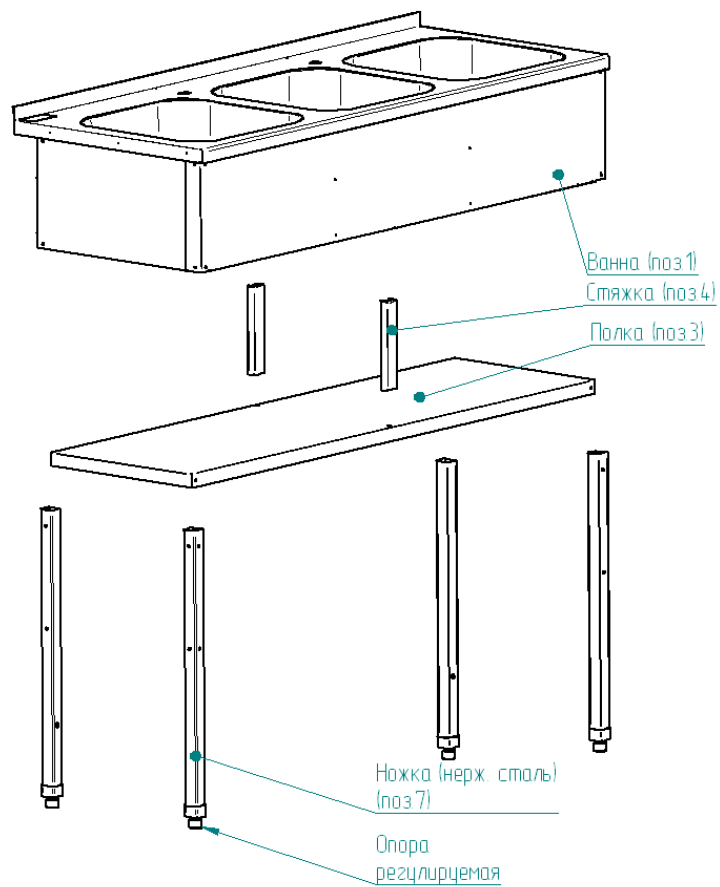
Рис.2 Сборка ванны с полкой
